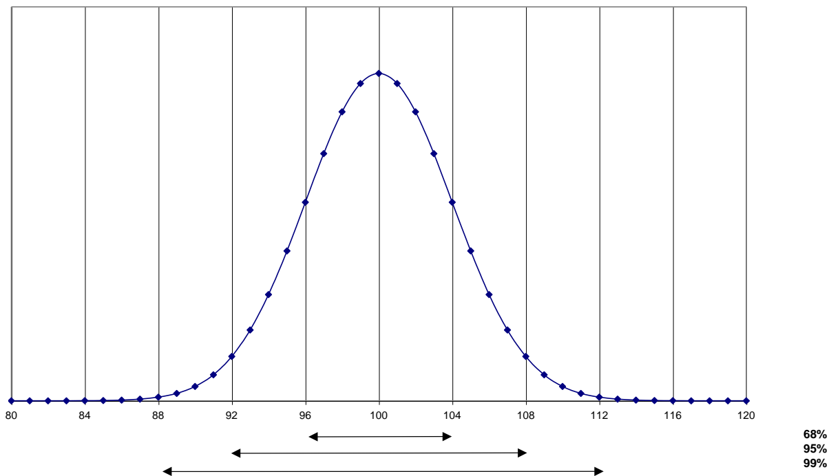
Figuur 2. Normale verdeling van fokwaarde met gemiddelde 100 en spreiding 4
