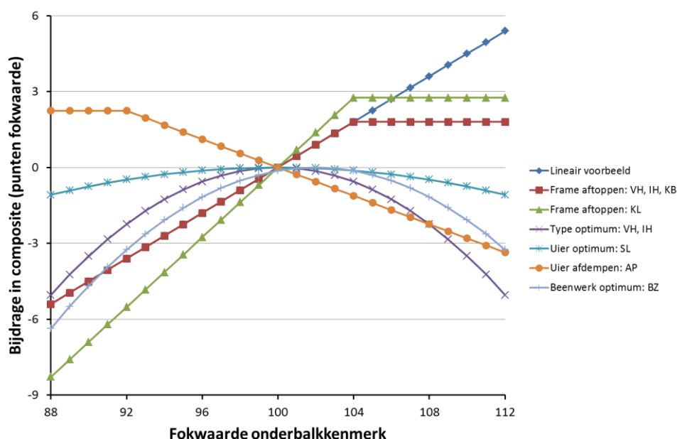
Figuur 1. Bijdrage in de composites voor melkdoel voor onderbalkkenmerken die lineair worden ingewogen, worden afgetopt, worden afgedempt, of als kwadratisch optimum worden ingewogen.
